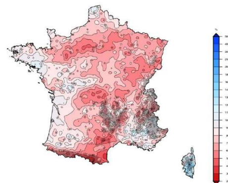
Rapport à la moyenne saisonnière de référence 1991-2020 des cumuls des précipitations France Hiver 2023
